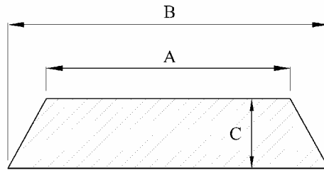
شکل ۸-۴- ابعاد ریسه
